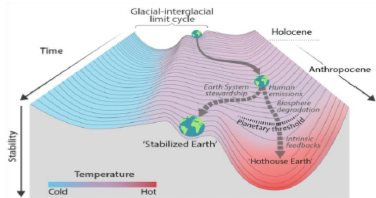
Gambar 1. Trajektori Bumi di Era Antroposen
