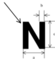
Gambar 1.c BENTUK DAN UKURAN HURUF ANGKUTAN LINTAS BATAS NEGARA
