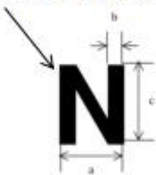
Gambar 3.c BENTUK DAN UKURAN HURUF ANGKUTAN ANTARKOTA DALAM PROVINSI
