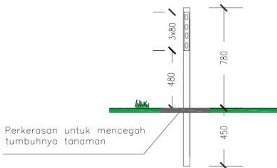
Gambar 24. Pagar Pengaman Fleksibel Dengan Empat Kabel
