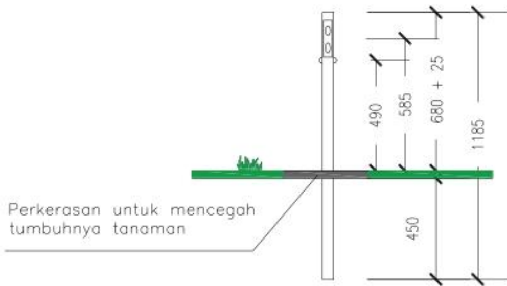
Gambar 23. Tipikal Penampang Melintang Pagar Pengaman Fleksibel
