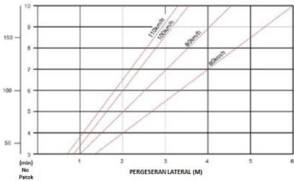
Gambar 42. Jarak Pemasangan Delineator Jalur Transisi
