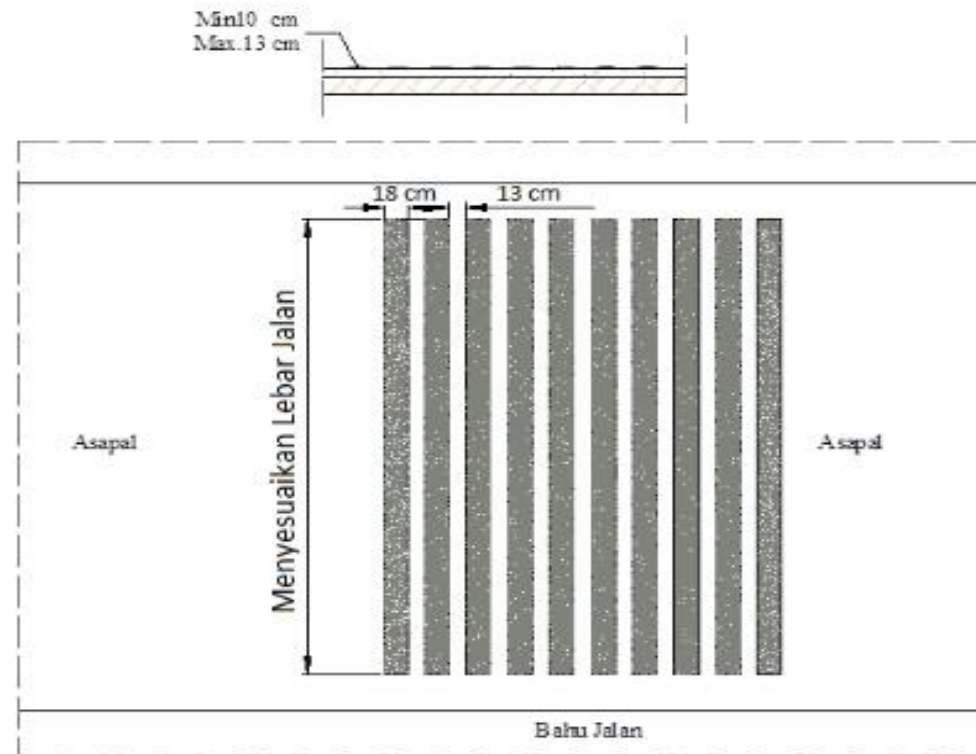
Gambar 57. Penampang melintang dan Membujur Pita Penggaduh Rumble Area
