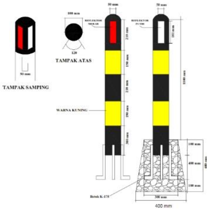
Gambar 44. Spesifikasi Delineator Pipa Besi
