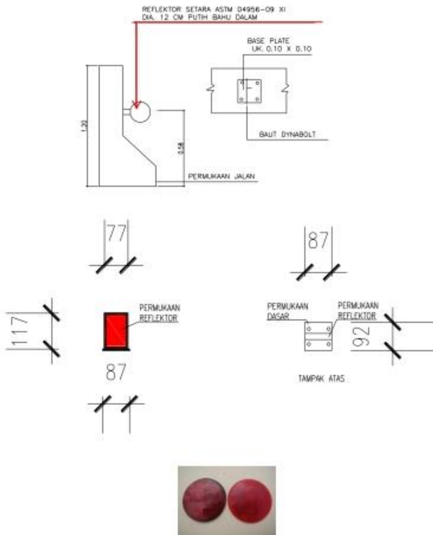
Gambar 9. Penempatan Reflektor Pada Pagar Pengaman Kaku
