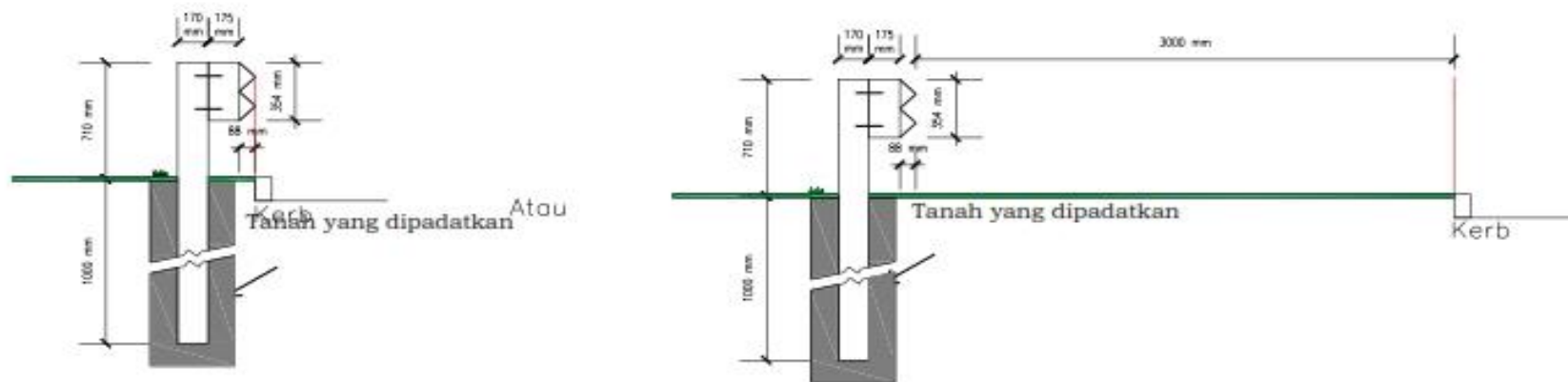
Gambar 11. Pagar Pengaman Semi Kaku Pada Jalan Kecepatan Rendah
