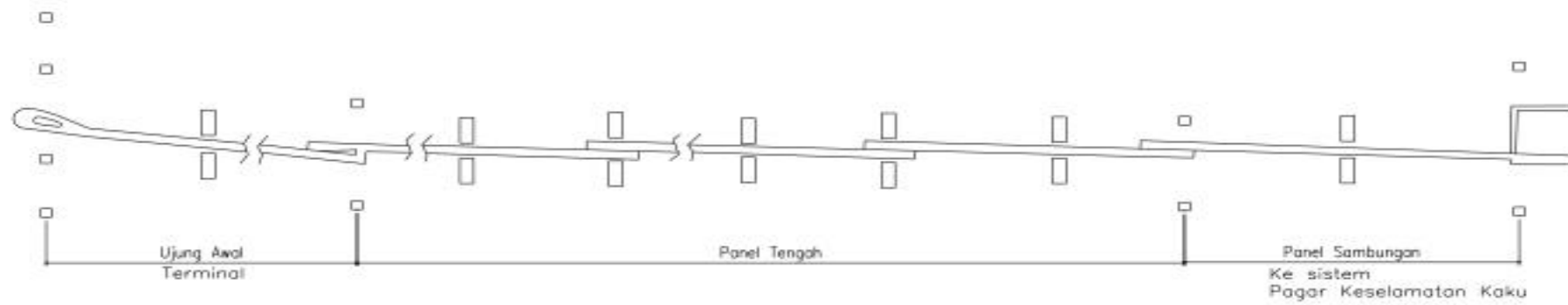
Gambar 15. Sambungan Pagar Pengaman Semi Kaku Sisi Jalan ke Sistem Pagar Pengaman Kaku
