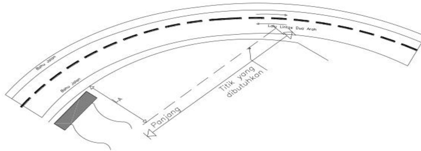
Gambar 18. Kebutuhan Pajang Pagar Pengaman Pada Sisi Dalam Tikungan
