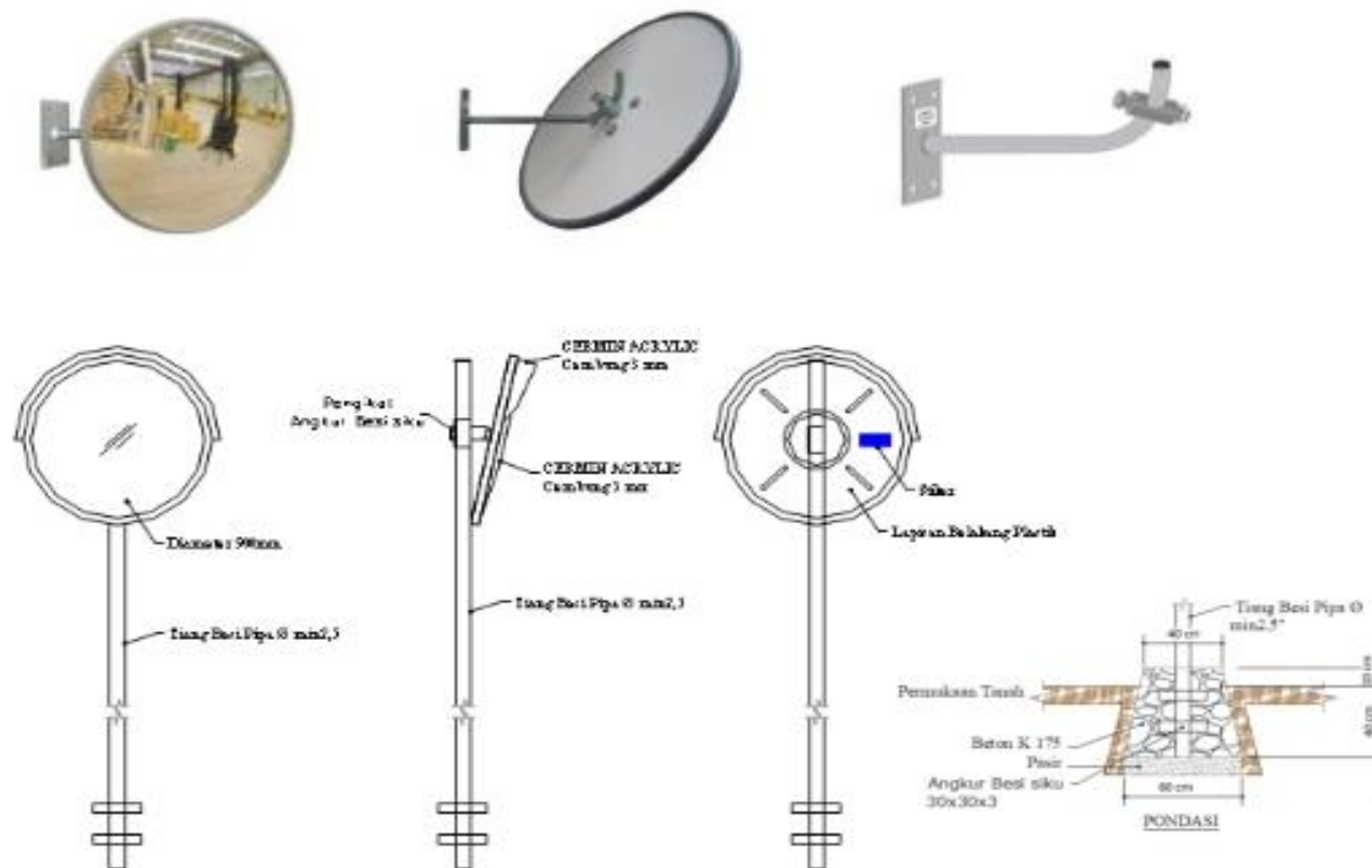
Gambar 37. Konstruksi Cermin Tikungan Lingkaran Penuh
