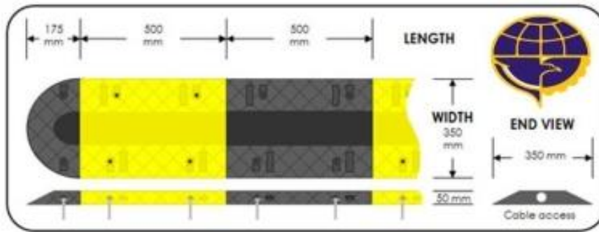
Gambar 2. Speed Hump dengan Uk : 350 x 50 mm
