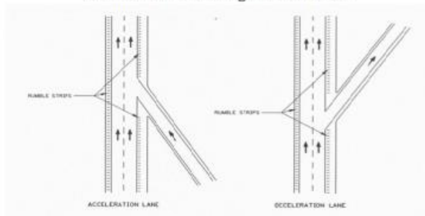
Gambar 52. Pemasangan Rumble Area
