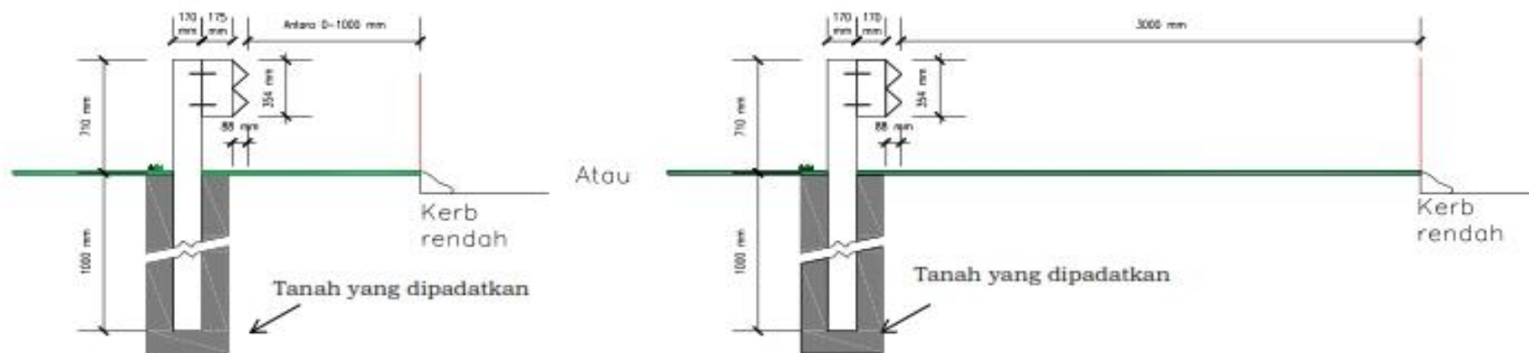
Gambar 12. Pagar Pengaman Semi Kaku Pada Jalan Kecepatan Tinggi
