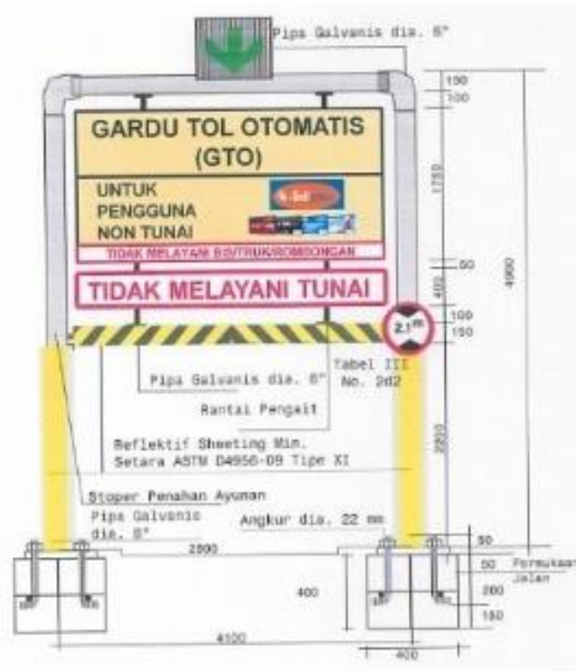
Gambar 4. Alat Pembatas Tinggi dan Lebar
