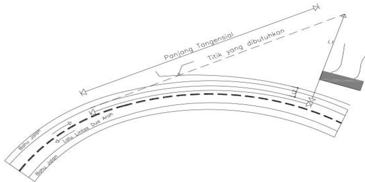
Gambar 17. Kebutuhan Pajang Pagar Pengaman Pada Sisi Luar Tikungan
