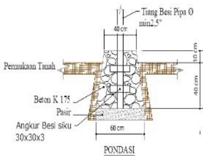
Gambar 36. Desain Pondasi Cermin Tikungan
