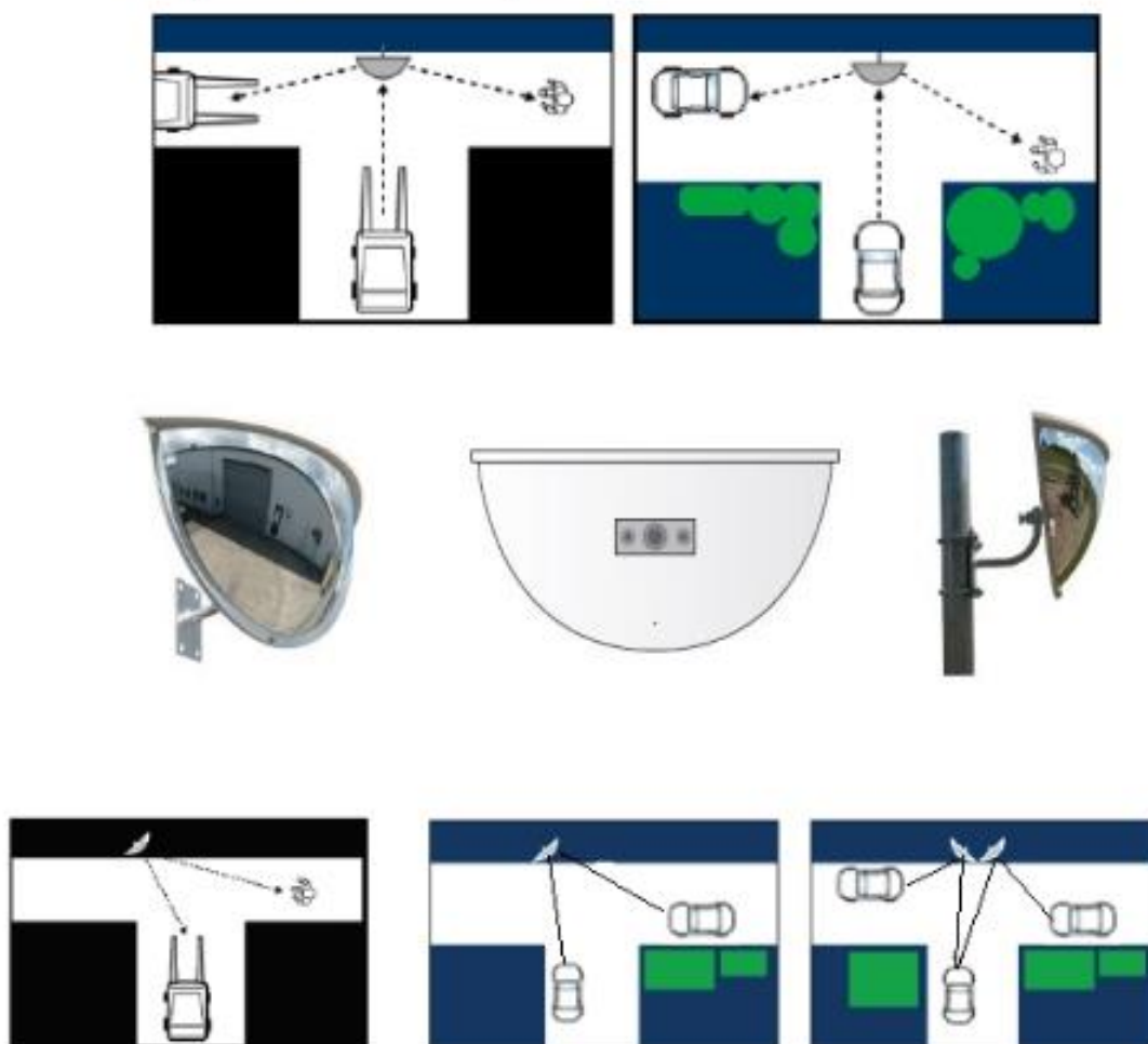
Gambar 35. Pemasangan Cermin Tikungan Lingkaran Penuh
