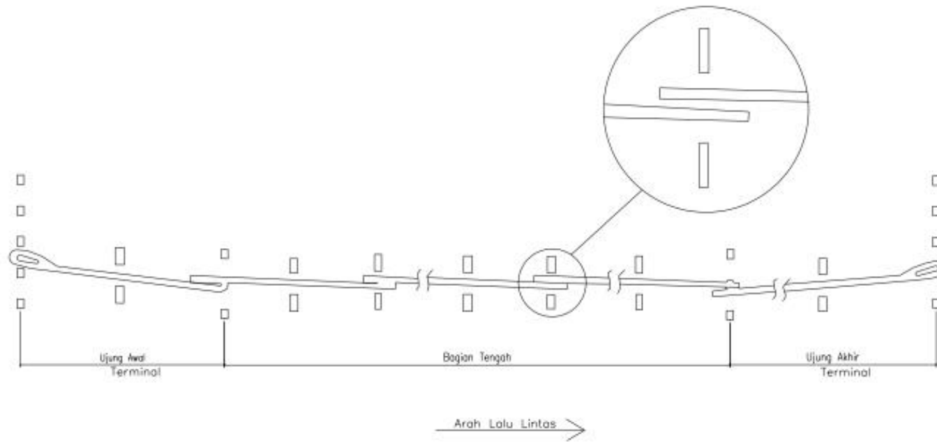
Gambar 14. Metode Penyambungan Beam tampak atas
