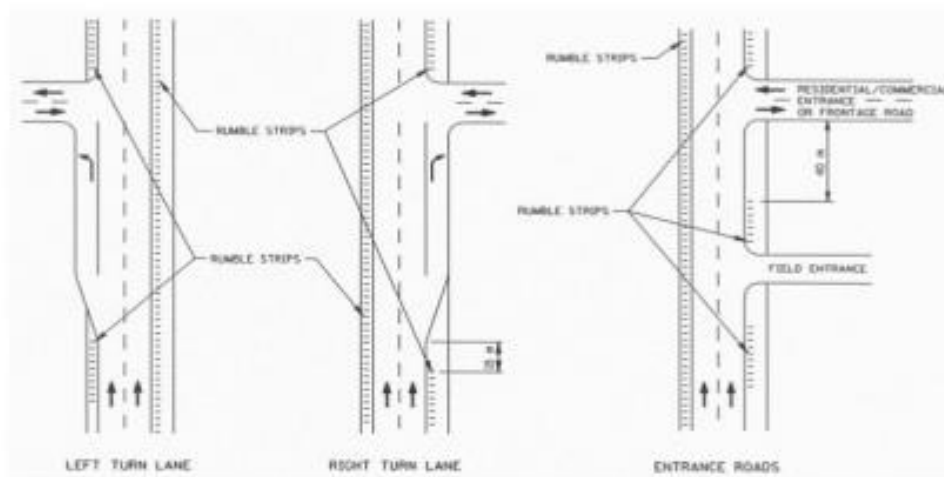
Gambar 53. Penempatan Soulder rumble
