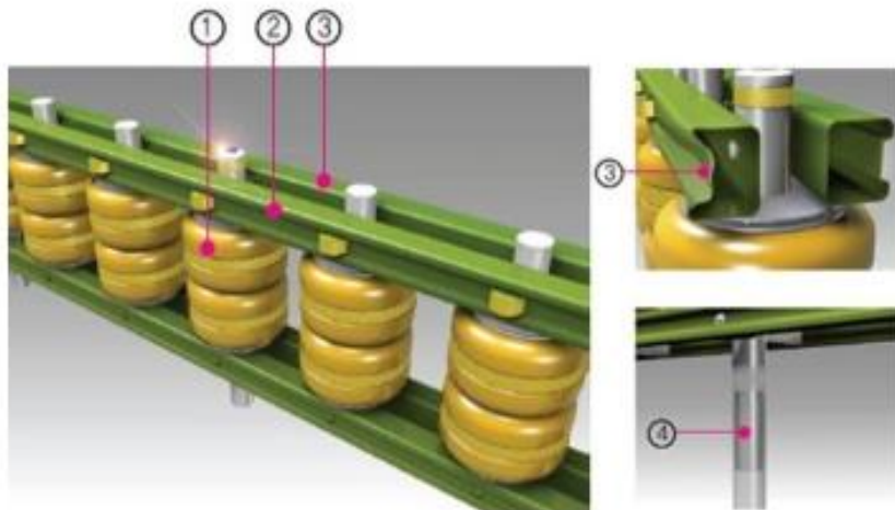
Gambar 29. Komponen Utama Safety Roller
