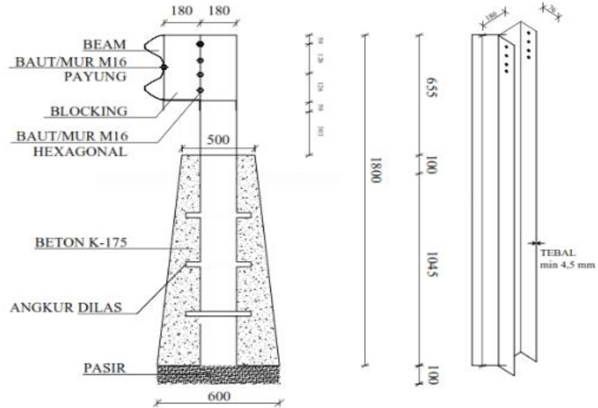
Gambar 21. Detail Desain Pondasi Post Jenis Beton Cor Pagar Pengaman Semi Kaku
