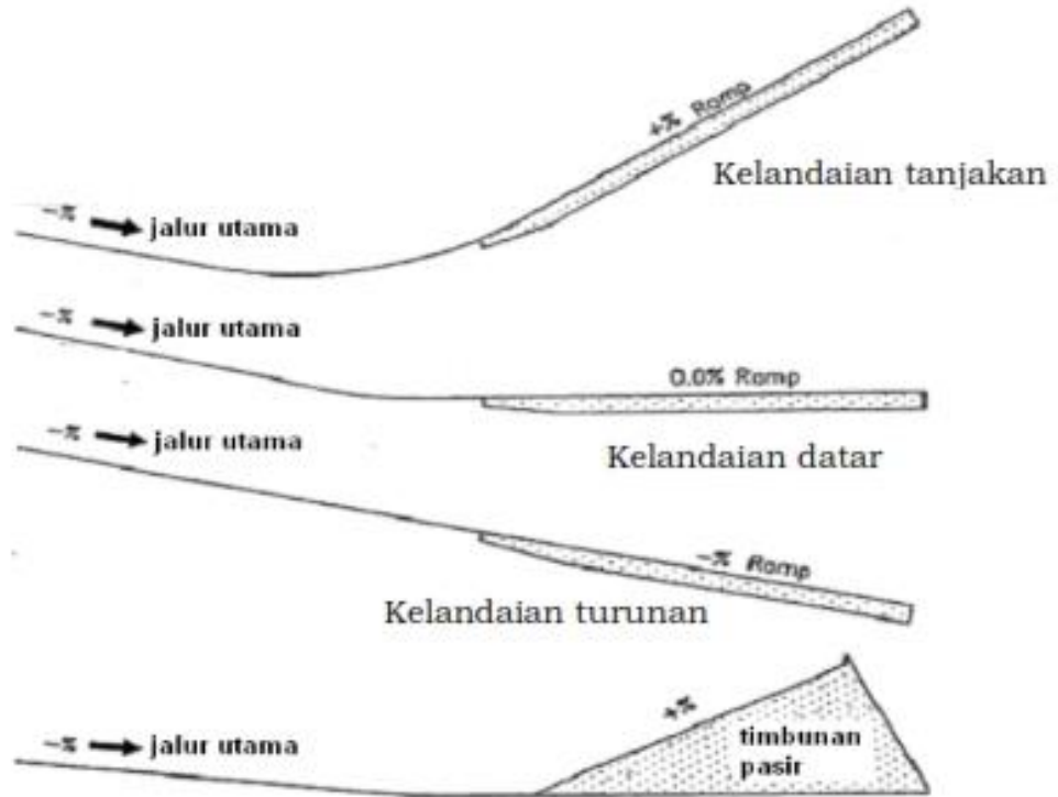
Gambar 58. Jenis Jalur Penghentian Darurat
