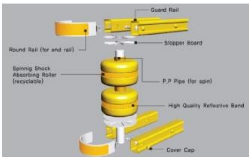
Gambar 31. Uraian Komponen Utama Safety Roller
