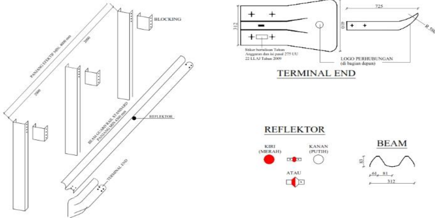
Gambar 20. Uraian komponen Utama Pagar Pengaman Semi Kaku
