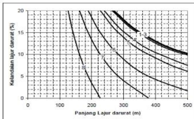
Gambar 60. Panjang Lajur Darurat Untuk Kecepatan Masuk 120 km/jam (Angka menunjukkan jenis material)
