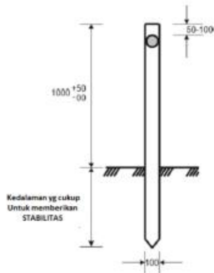
Gambar 44. Spesifikasi Delineator Pipa Besi
