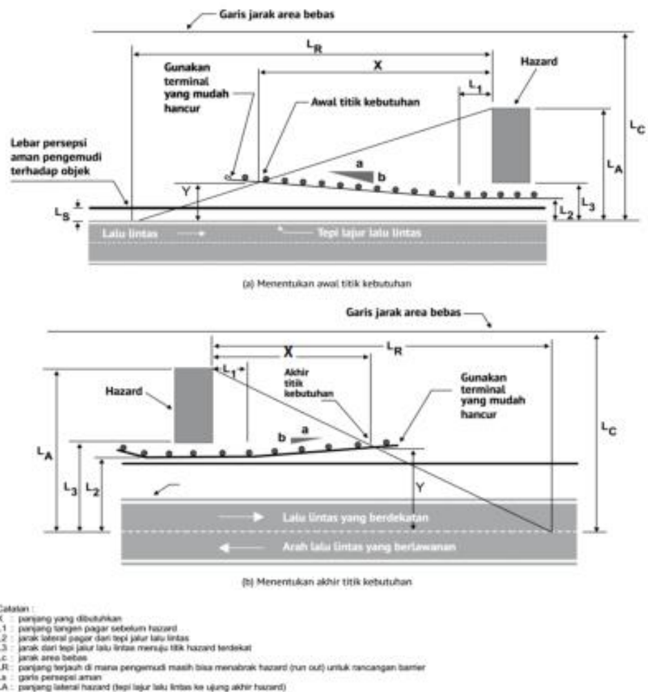
Gambar 16. Panjang Kebutuhan Pagar Pengaman Pada Sisi Jalan Lurus
