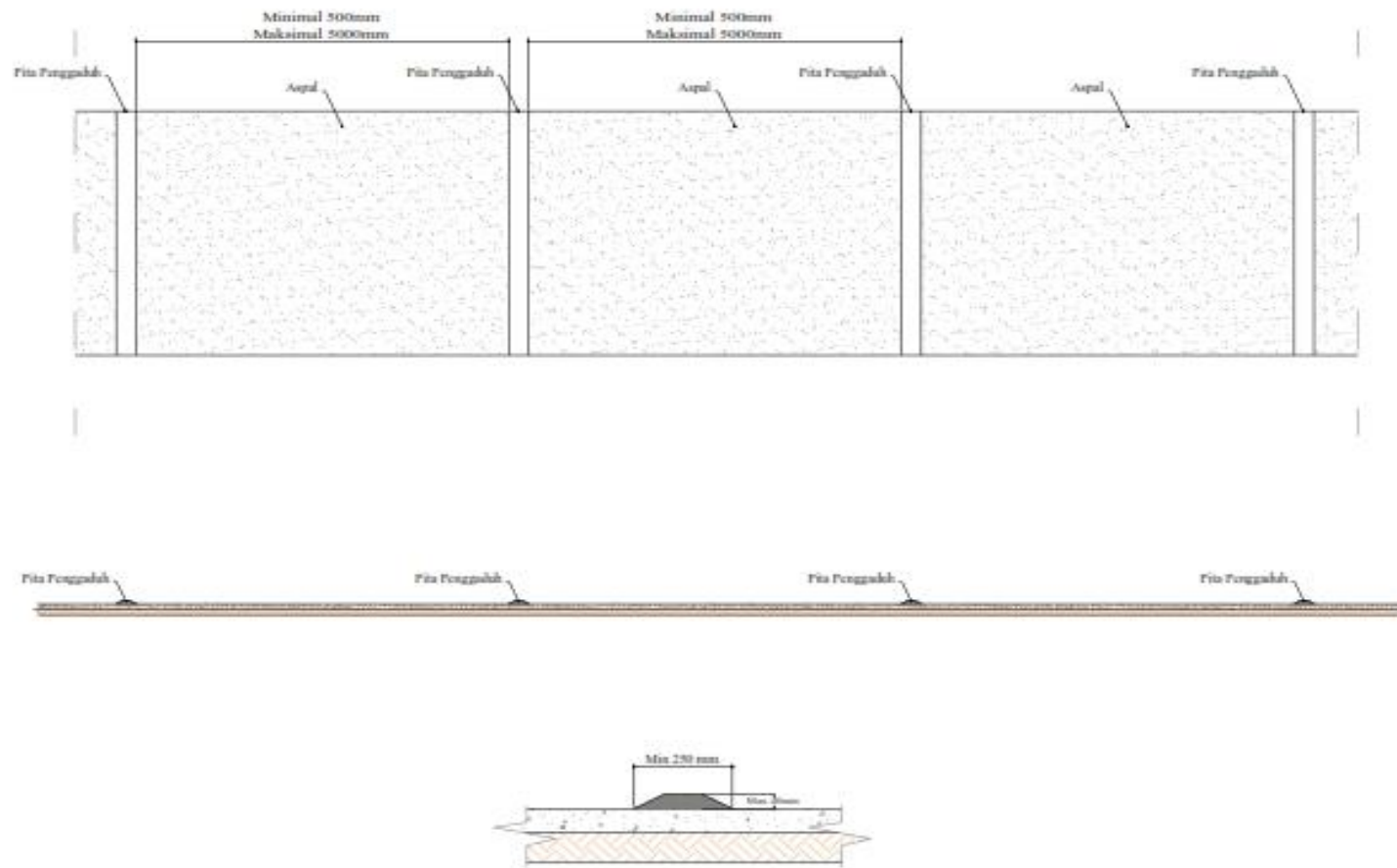
Gambar 54. Penampang melintang dan Membujur Pita Penggaduh Rumble Strip
