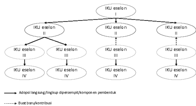
Gambar 34. Pohon IKU
