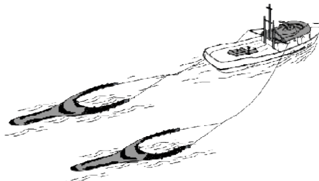
Gambar 5. Pukat udang
