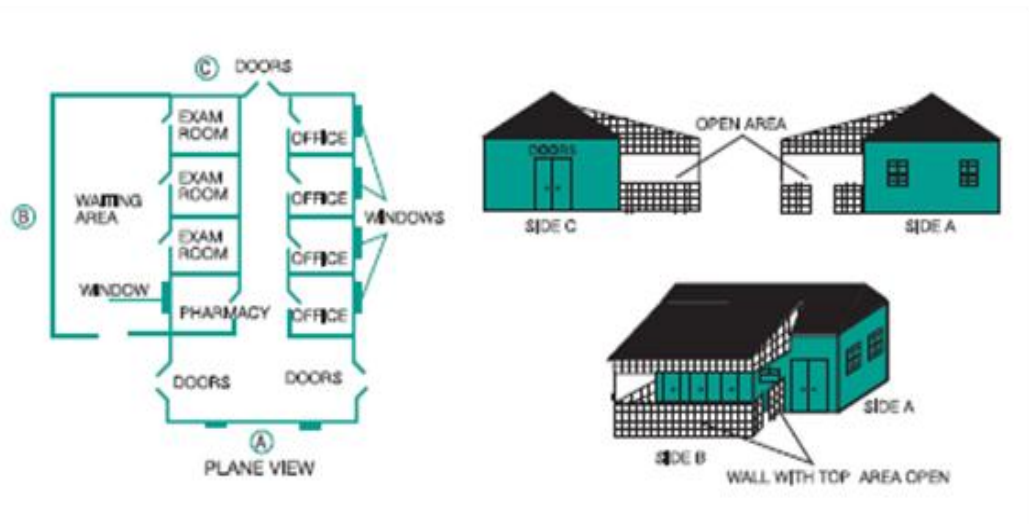
Gambar 23. Ruang tunggu yang memanfaatkan ventilasi alami
