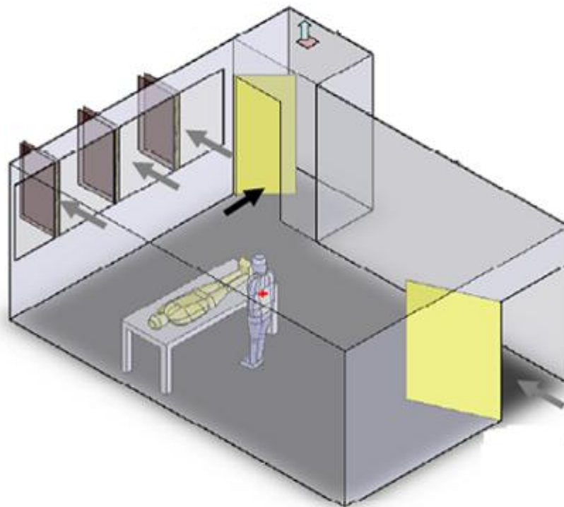
Gambar 32. Perhitungan Laju Pertukaran Udara
